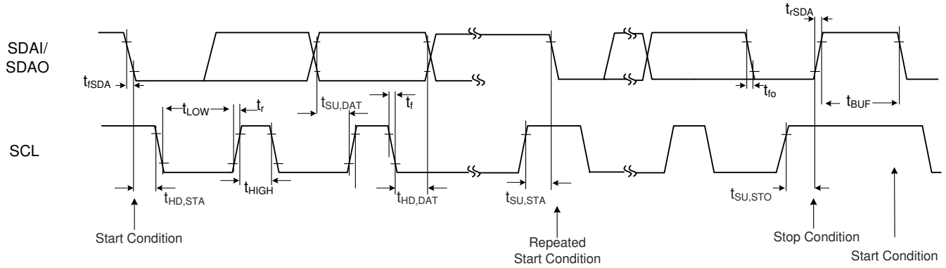
图 8-1. I 2 C Timings
