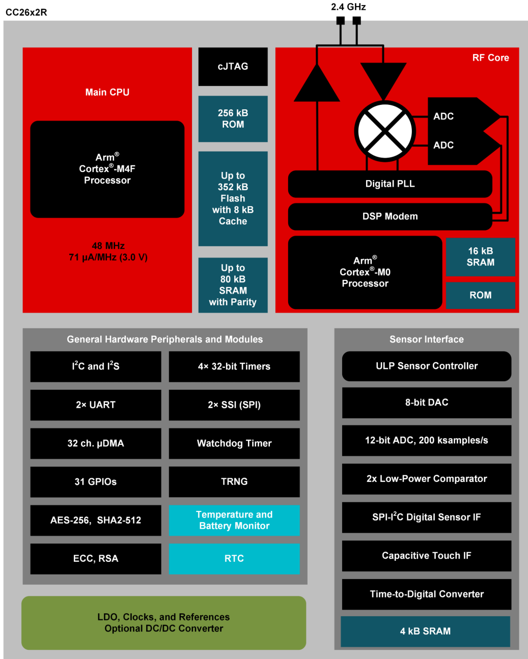
图 4-1. CC2652R 方框图
