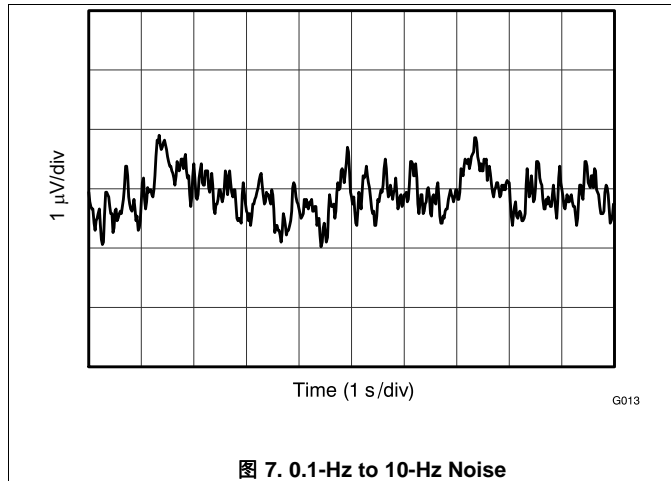
图 7. 0.1-Hz to 10-Hz Noise
