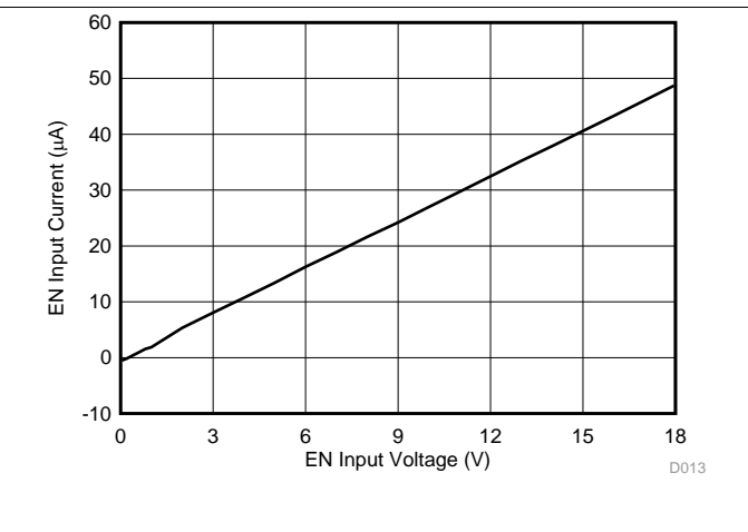
Figure 13. EN Current vs EN Voltage
