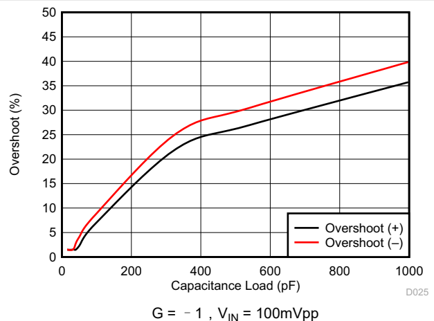
图 6-20. 小信号过冲与容性负载间的关系
