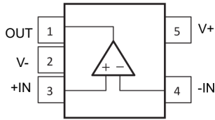
图 5-1. LMV321A DBV 封装，5 引脚 SOT-23 (顶视图)
