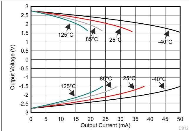
图 6-7. 输出电压与输出电流间的关系 (爪形)
