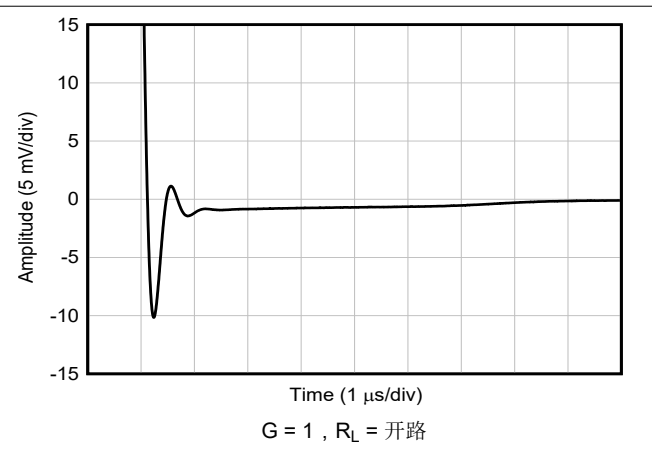
图 5-28. 大信号阶跃响应 (下降)
