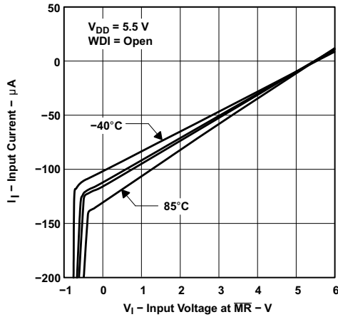
图 7-4. MR 处的输入电流与输入电压间的关系
