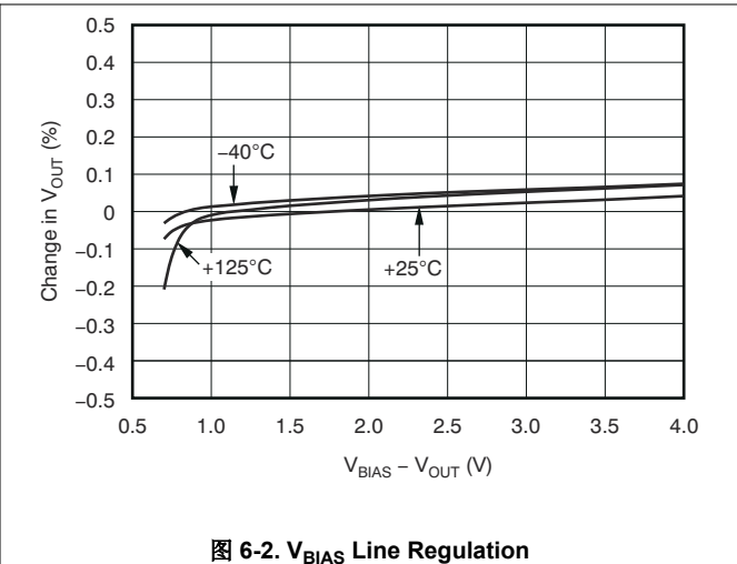
图 6-2. V_{BIAS} Line Regulation
