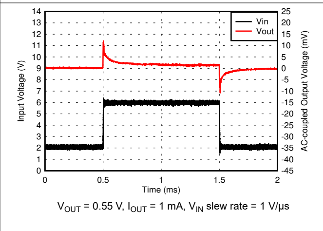
图 6-24. 0.55-V Line Transient
