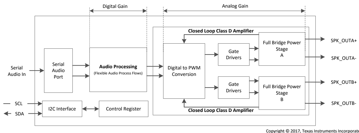
图 7-7. Speaker Amplifier Gain
