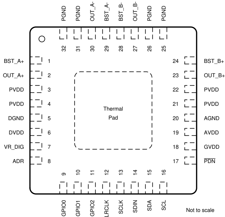
图 5-1. RHB Package 32-Pin VQFN
