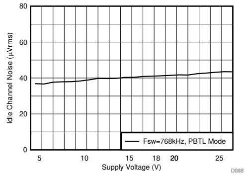
A. BD Modulation F_{SW} = 768 \text{ kHz} \text{Load} = 4 \Omega PBTL Mode
