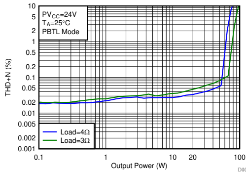
图 8-10. THD+N vs Output Power
