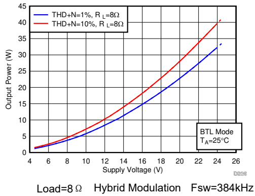
图 8-2. Output Power vs PVDD
