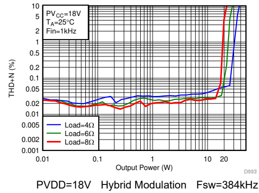
图 8-7. THD+N vs Power
