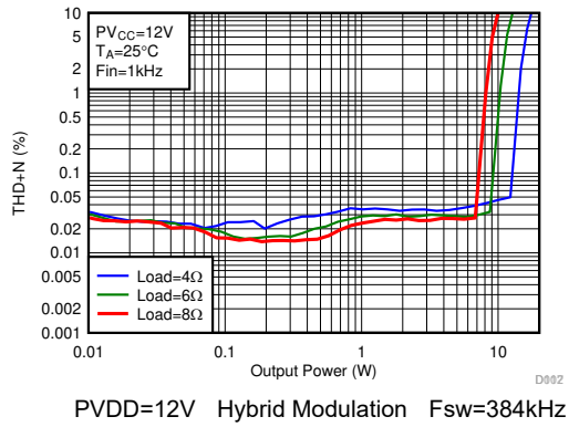
图 8-6. THD+N vs Power
