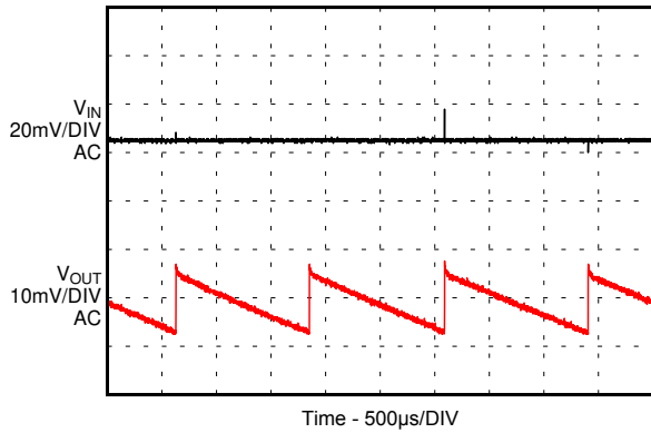
Time - 500µs/DIV
