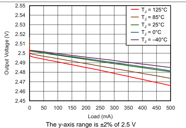
图 4. TPS735 Load Regulation
