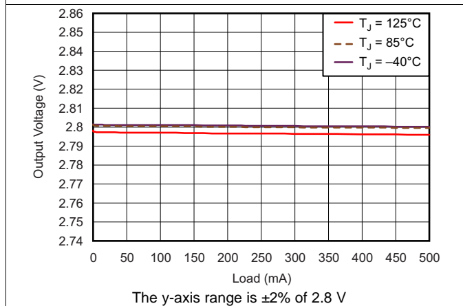
图 3. TPS735 Load Regulation
