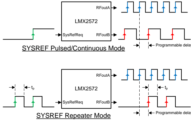
图 35. SYSREF Modes
