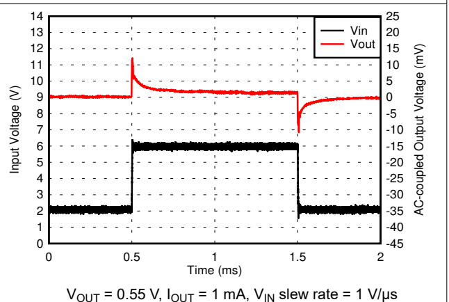
图 6-30. 0.55-V Line Transient
