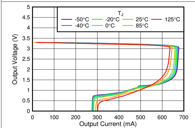
图 6-29. 3.3-V V_{OUT} vs I_{OUT}
