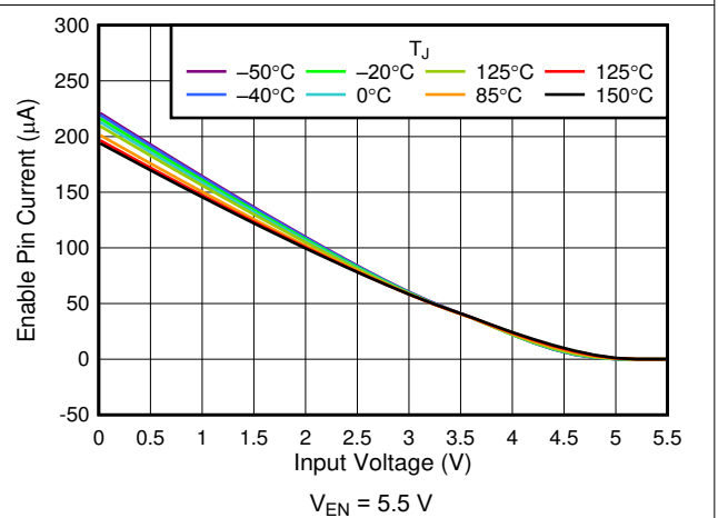
图 6-28. I_{EN} vs V_{IN}
