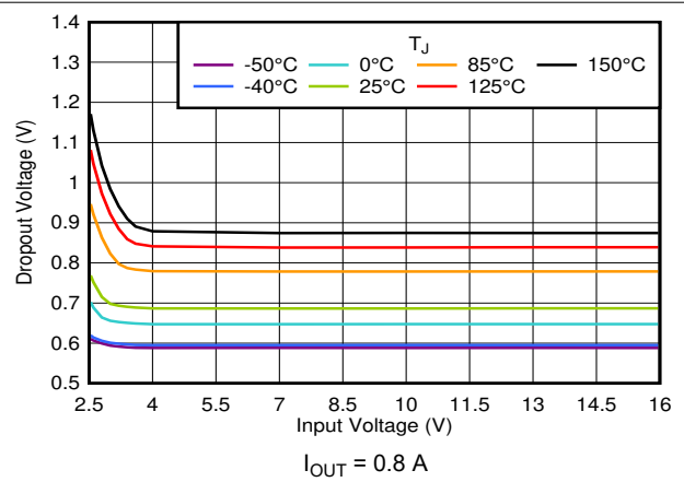
图 7-16. V_{DO} vs V_{IN}
