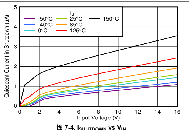
图 7-4. I_{SHUTDOWN} vs V_{IN}
