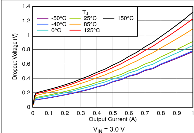
图 7-17. V_{DO} vs I_{OUT}
