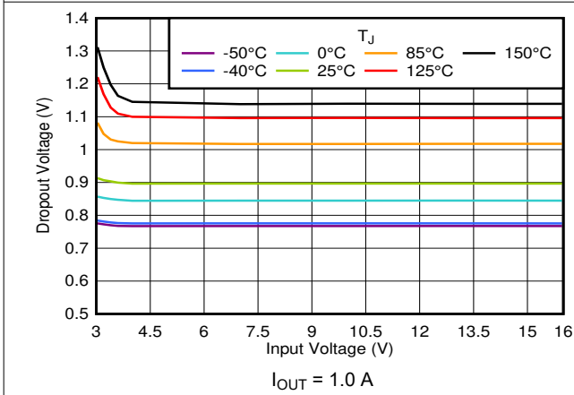
图 7-15. V_{DO} vs V_{IN}
