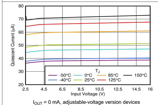
图 7-5. I_Q vs V_{IN}
