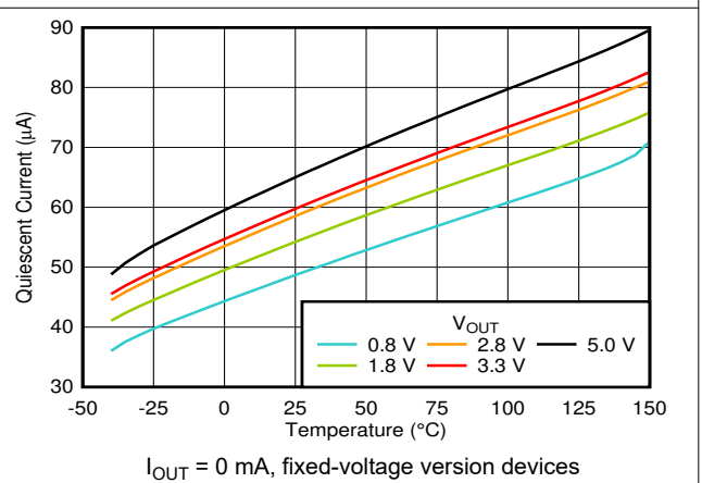
图 7-6. I_Q vs Temperature
