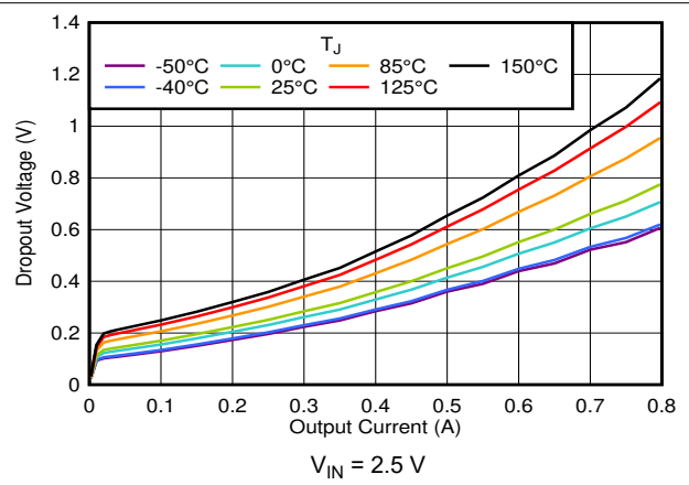
图 7-18. V_{DO} vs I_{OUT}
