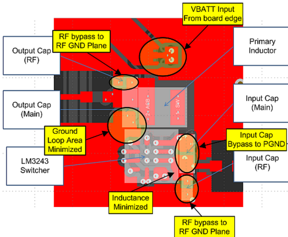
Figure 29. Top Layer
