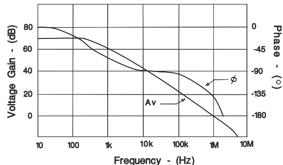
图 6-2. 误差放大器开环频率响应
