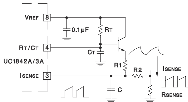
图 7-7. 斜率补偿
