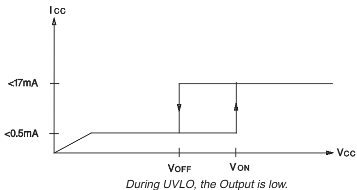
图 7-3. 欠压锁定
