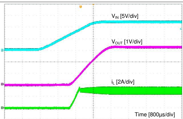
图 15. DCM Mode
