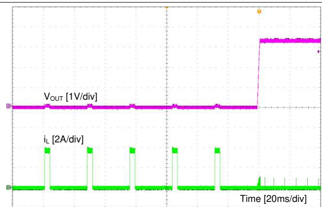
图 21. Short Recovery
