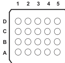
图 5-1. NME/GXY/ZXY 封装 (底视图)
