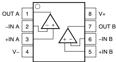
D、DGK 封装 8 引脚 MSOP、SO 俯视图
