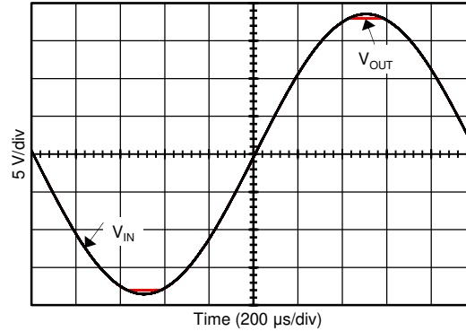
图 8-2. No Phase Reversal
