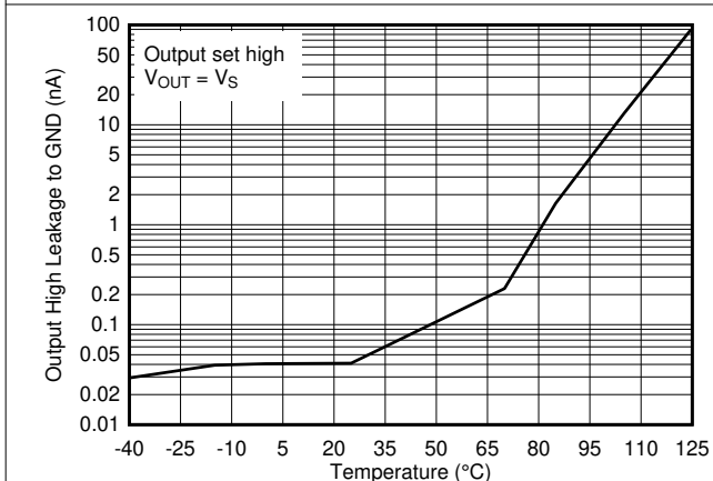
图 6-28. 5V 下输出高电平漏电流与温度之间的关系
