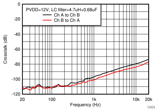
图 6-27. Crosstalk
