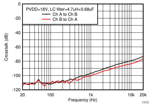
图 6-28. Crosstalk
