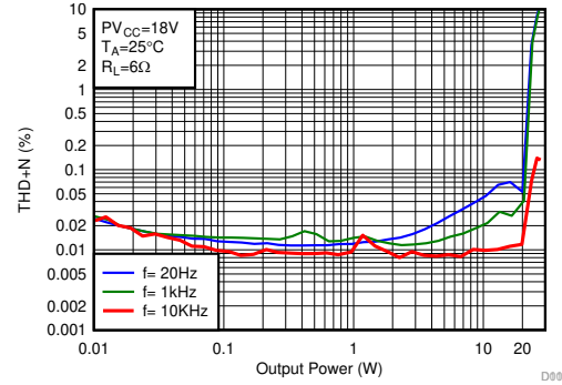
图 6-20. THD+N vs Output Power-BTL
