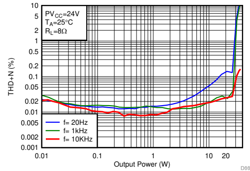
图 6-22. THD+N vs Output Power-BTL
