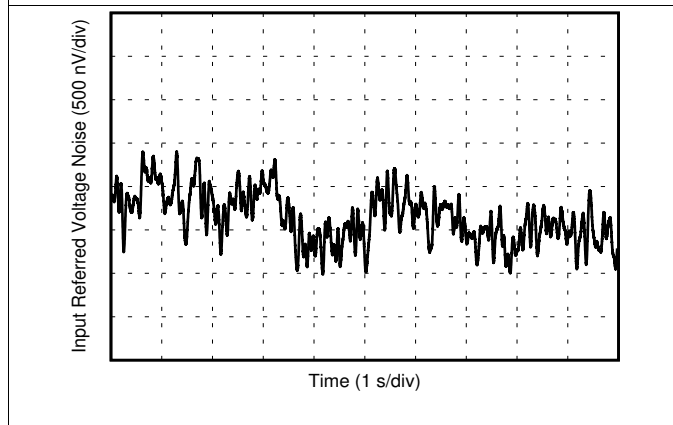
图 9. 0.1-Hz to 10-Hz Noise
