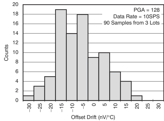
图 6-14. Offset Drift (25°C to 105°C)
