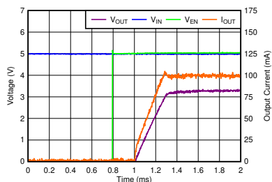
启动波形
