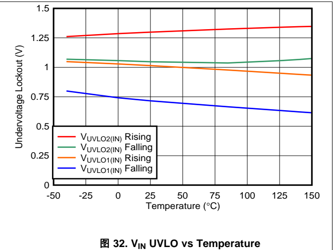
图 32. V_{IN} UVLO vs Temperature
