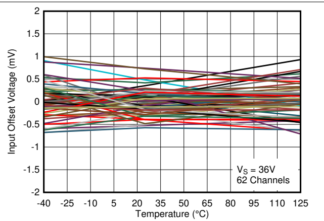
图 6-15. 36V 下输入失调电压与温度之间的关系
