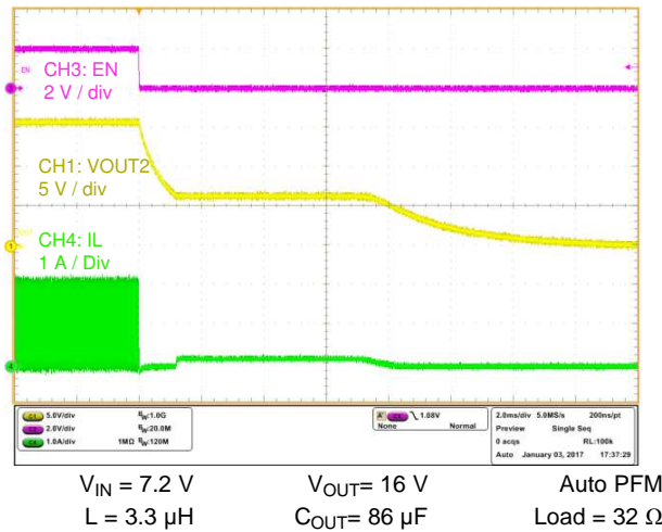
图 29. Shutdown by EN
