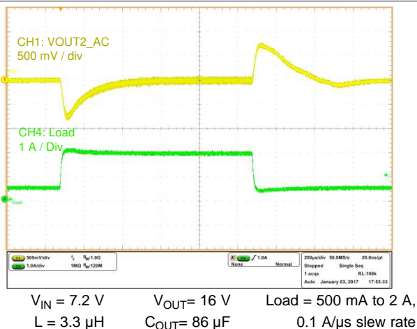
图 30. Load Transient
