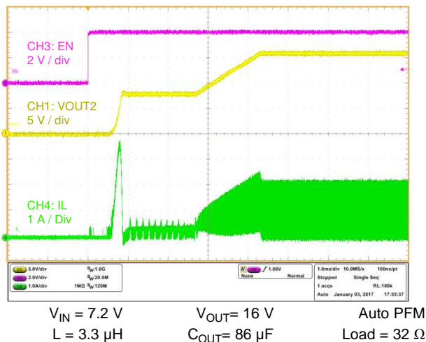
图 28. Startup by EN
