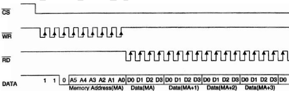
READ 模式 (读连续地址)
