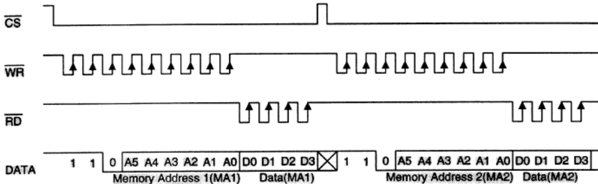
READ 模式 (命令代码110)
