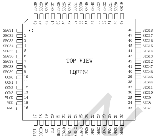
TM1729-LQFP64
