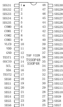
TM1729-TSSOP48/SSOP48
