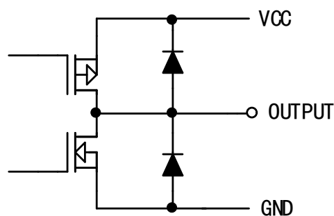
输出管脚
