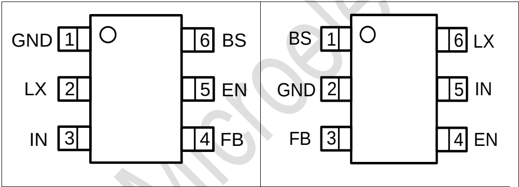
SOT23-6
