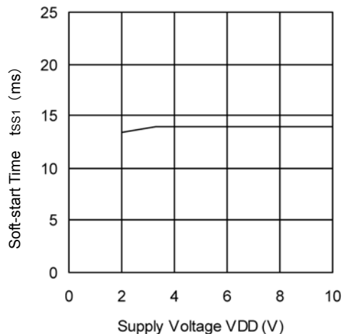
XC9505B092 (180kHz)
