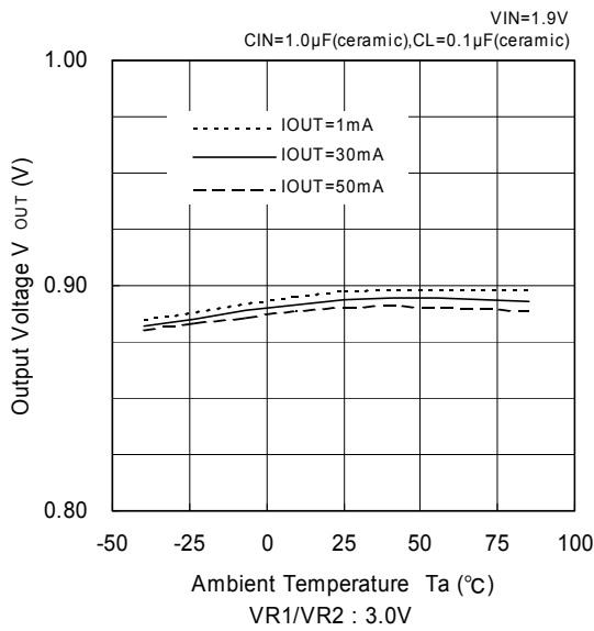
VR1/VR2 : 3.0V
