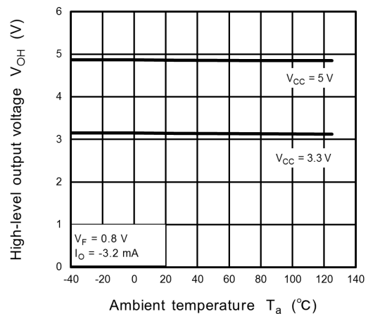
Fig. 13.2.6 V_{OH} - T_a
