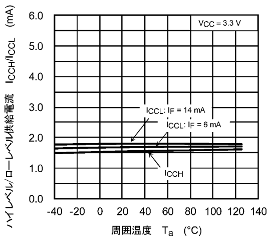
図 12.2.5 I_{CCH}/I_{CCL} - T_a
