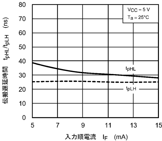
図 12.2.15 t_{pHL}/t_{pLH} - I_F
