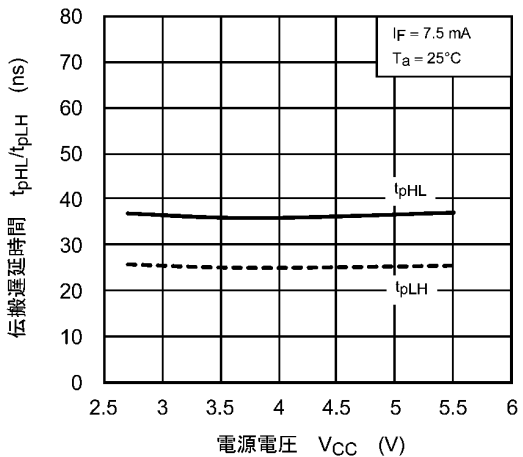
図 12.2.17 t_{pHL}/t_{pLH} - V_{CC}
