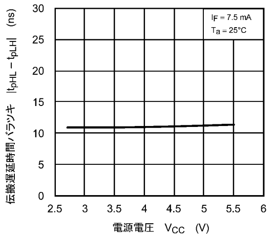
図 12.2.18 |t_{pHL} - t_{pLH}| - V_{CC}
