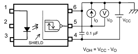
Fig. 12.1.2 VOH Test Circuit
