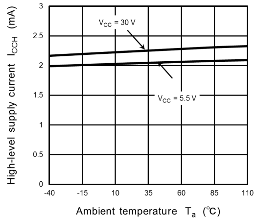
Fig. 12.2.8 I_{cCH} - T_a
