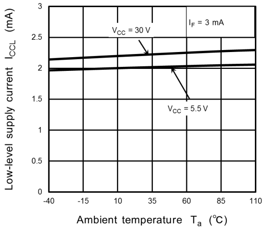
Fig. 12.2.7 I_{cCL} - T_a
