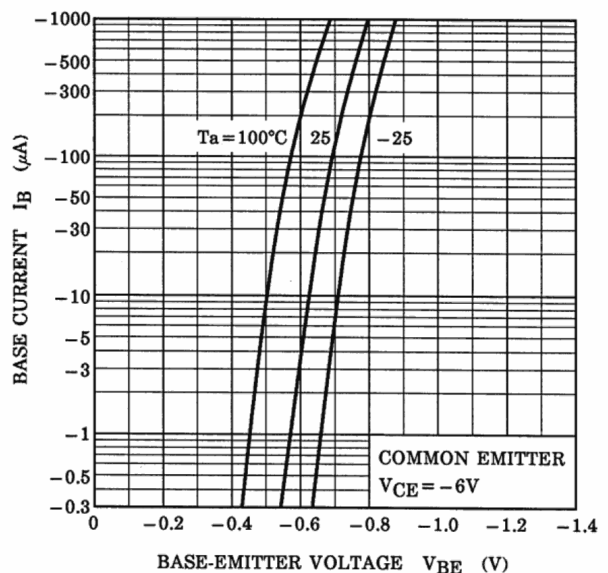
Fig. 14.6 I_B - V_{BE}
