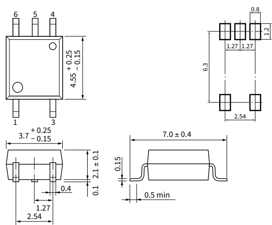
5 pin SO6
