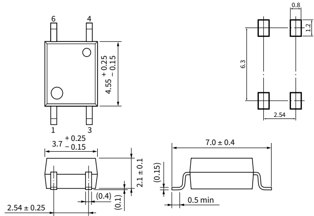
4 pin SO6
