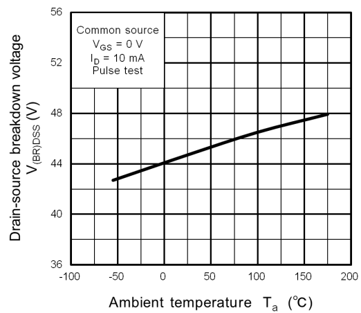
Fig. 8.12 V_{(BR)DSS} - T_a
