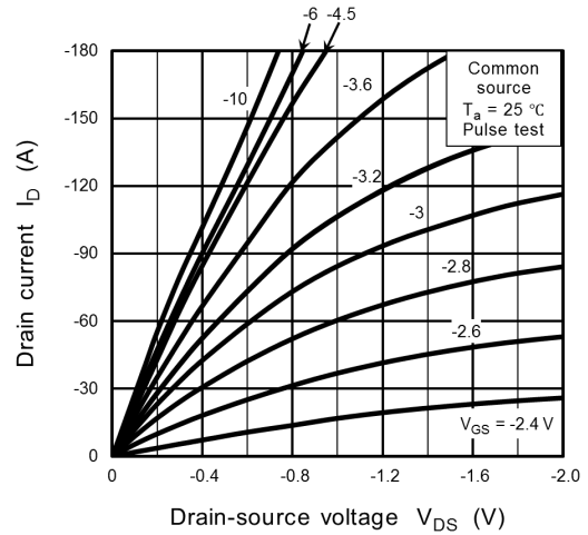
Fig. 8.2 I_D - V_{DS}
