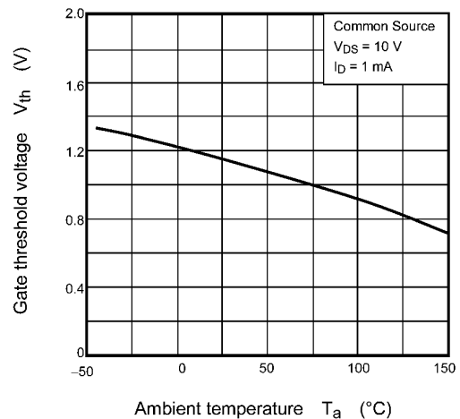
Fig. 7.6 V_{th} - T_a
