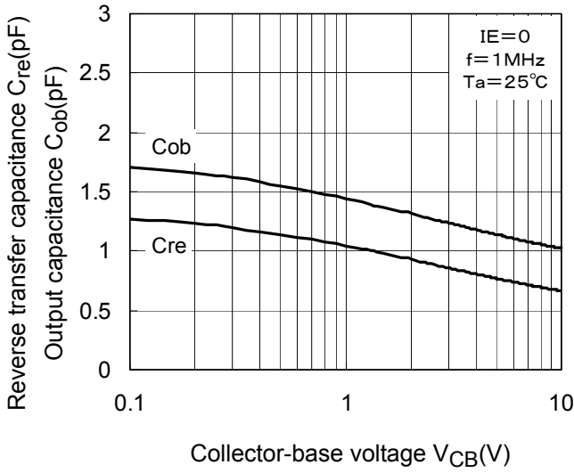
C_{re}, C_{ob}-V_{CB}
