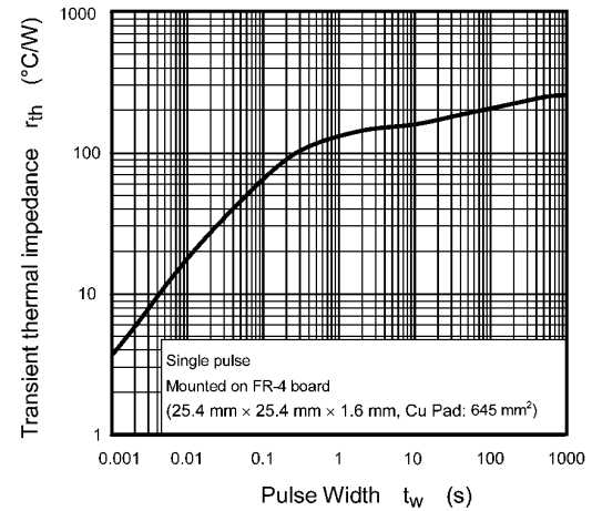
Fig. 7.12 r_{th} - t_w
