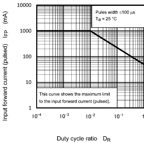
Fig. 11.3 I_{FP} - D_R
