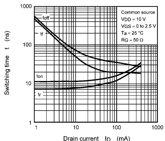
Fig. 8.10 t - I_D
