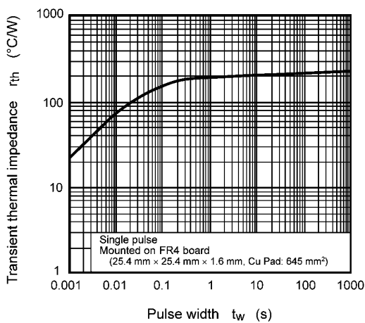
Fig. 8.11 r_{th} - t_w
