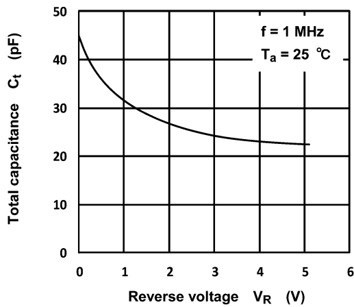
Fig. 7.3 C_t - V_R
