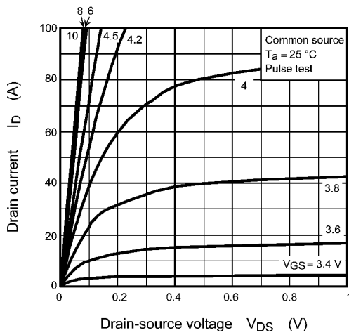
Fig. 9.1 I_D - V_{DS}
