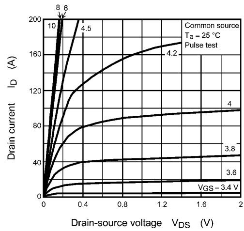
Fig. 9.2 I_D - V_{DS}
