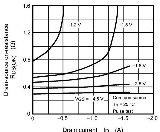
Fig. 8.6 R_{DS(ON)} - I_D
